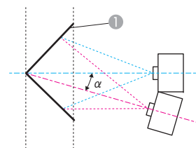
Vue supérieure
